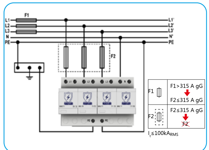
Paralel Bağlantı
